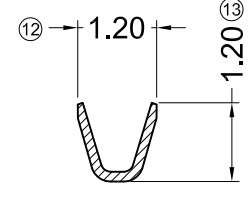
SECTION: B-B SCALE: 1:1
